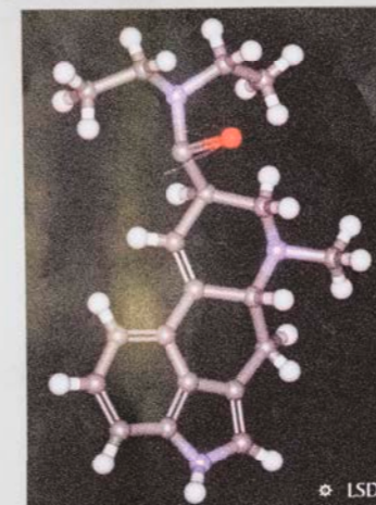
FORMULE MOLÉCULAIRE DU LSD
